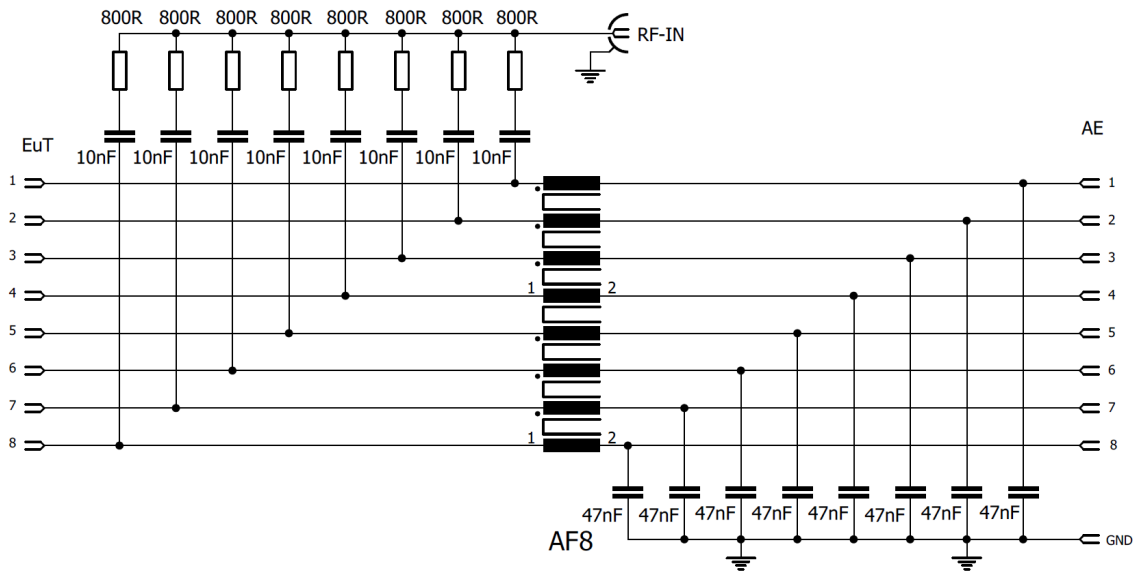
Bild 5: Prinzipschaltbild CDN AF8 Fig. 5: principal circuitry CDN AF8
