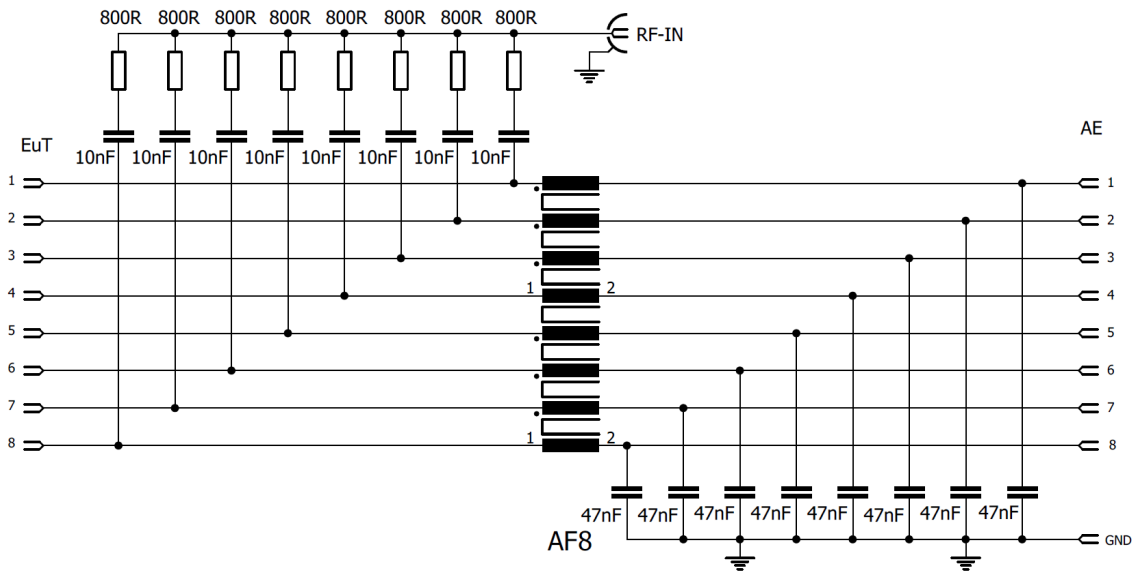
Bild 3: Prinzipschaltbild CDN AF8 Fig. 3: principal circuitry CDN AF8
