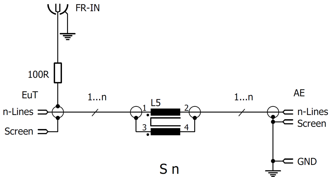
Bild 4: Prinzipschaltbild CDN S19 HDMI Fig. 4: principal circuitry CDN S19 HDMI
