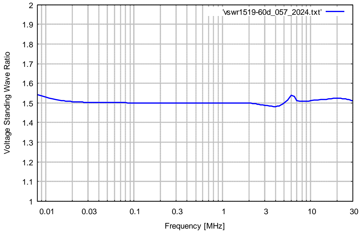
Spannungsstehwellenverhältniss (typ.)
