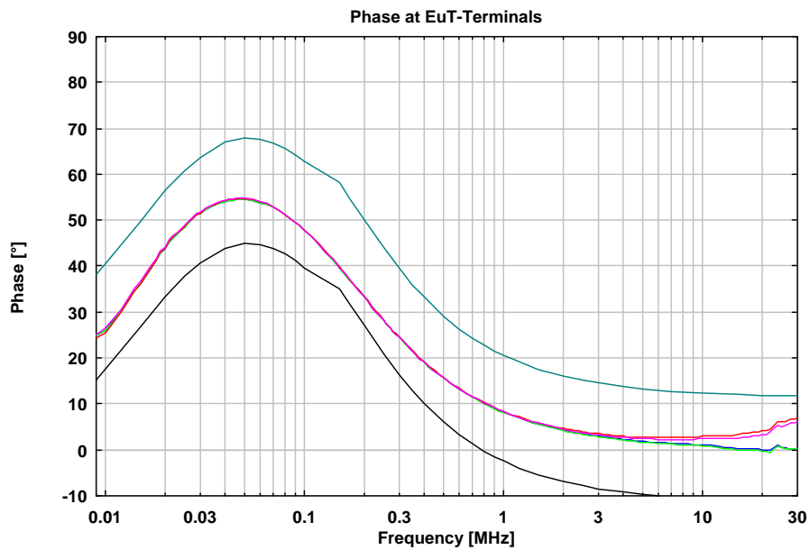
Abb. 5 Phase an den Prüflingsklemmen (CEKON), BNC mit 50 Ω Abschluss Phase at the connector for DuT (CEKON), BNC terminated with 50 Ω
