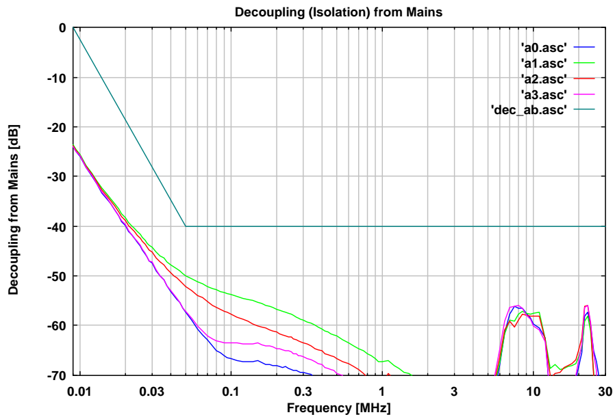
Abb. 9 Entkopplung vom Speisernetz (CEKON-Prüflingsklemmen), BNC mit 50 Ω Abschluss Decoupling from supply net (CEKON), BNC terminated with 50 Ω
