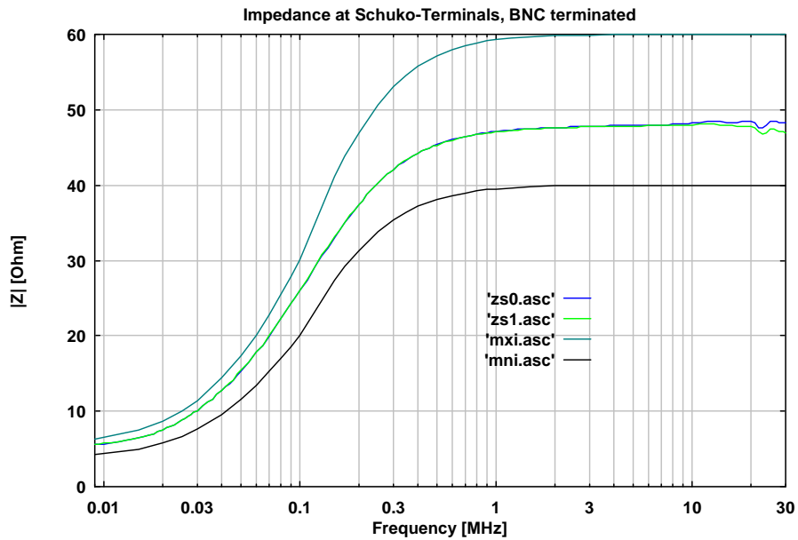
Abb. 7 Impedanz an den Prüflingsklemmen (SCHUKO), BNC mit 50 Ω Abschluss Impedance of connector for DuT (Schuko), BNC terminated with 50 Ω
