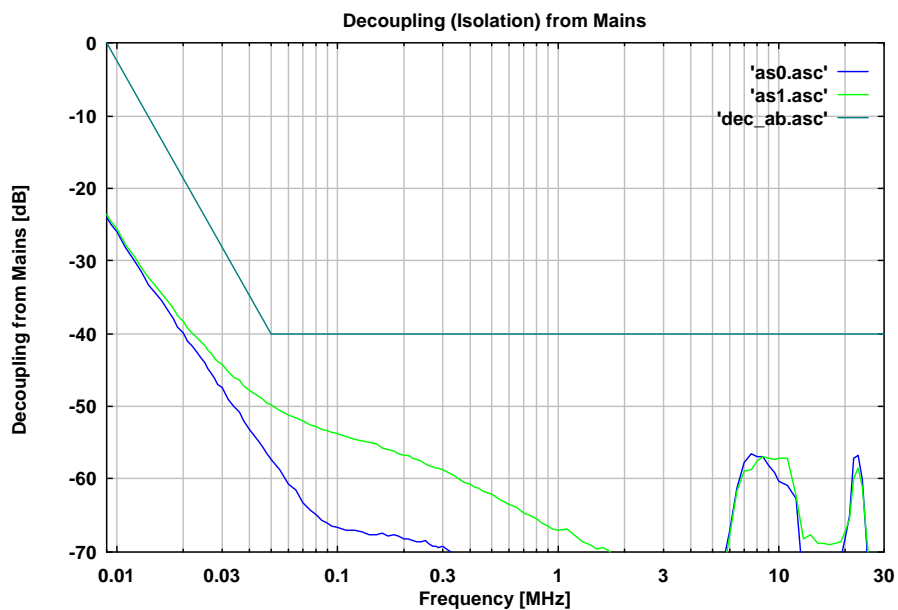
Abb. 10 Entkopplung vom Speisernetz (SCHUKO-Prüflingsklemmen), BNC mit 50 Ω Abschluss/ Decoupling from supply net (Schuko), BNC terminated with 50 Ω
