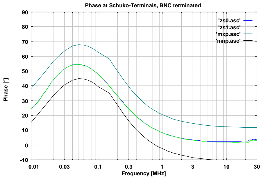
Abb. 8 Phase an den Prüflingsklemmen (SCHUKO), BNC mit 50 Ω Abschluss Phase at the connector for DuT (Schuko), BNC terminated with 50 Ω
