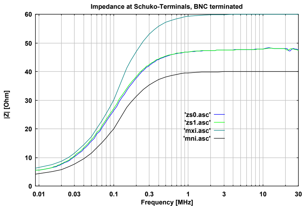
Abb. 4 Betrag der Impedanz an den Prüflingsklemmen, BNC mit 50 \Omega Abschluss Fig. 4 Magnitude of the impedance at the DuT connectors, BNC terminated with 50 \Omega
