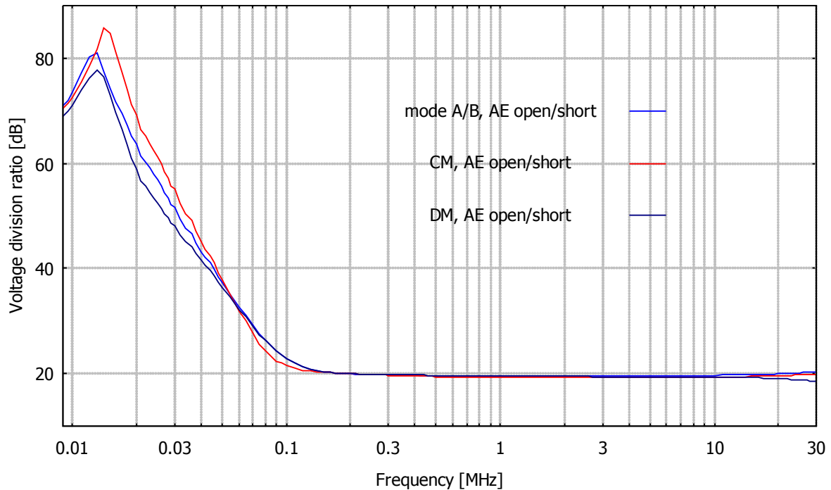
Entkopplung zwischen EuT und Speiseklemmen AE im 50 \Omega System (CM) und in 150 \Omega System (DM) Decoupling between EuT and Generator Terminals AE (50 \Omega System for CM and 150 \Omega system for DM)
