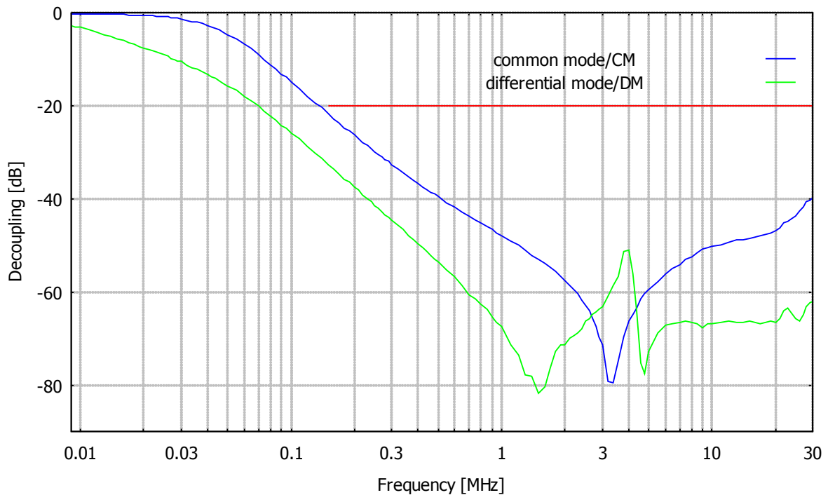
Entkopplung zwischen EuT und Speiseklemmen AE im 50 \Omega System (CM) und in 150 \Omega System (DM) Decoupling between EuT and Generator Terminals AE (50 \Omega System for CM and 150 \Omega system for DM)
