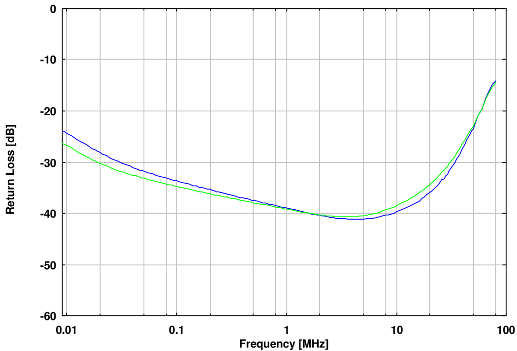
Abb. 2 Anpassung des SY9223-135 (EuT mit 135 \Omega abgeschlossen) Fig. 2: Return loss of SY9223-135 (EuT terminated with 135 \Omega )
