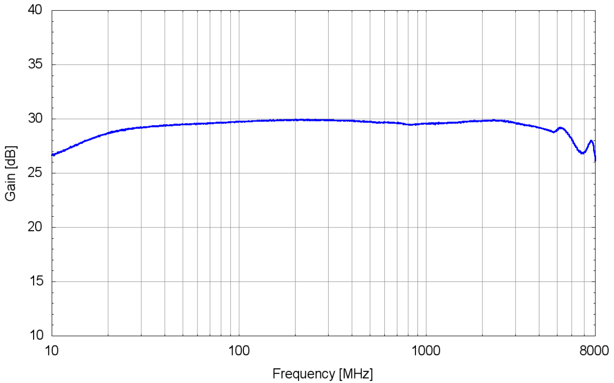
Verstärkung / Gain
